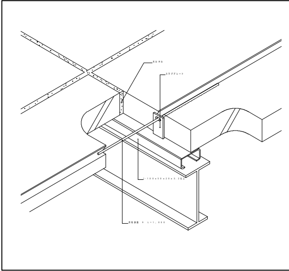
ヤネ1カP-2
