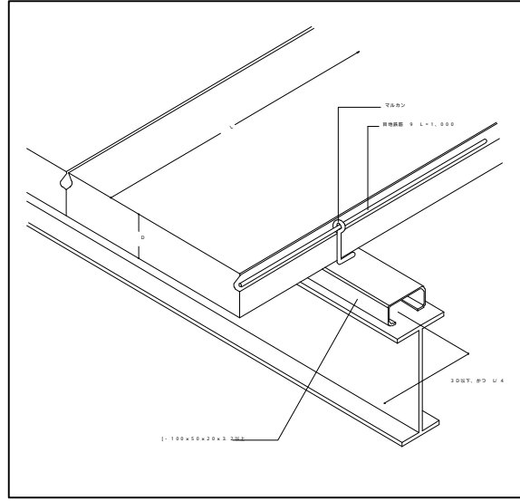
ヤネ1カP-9
