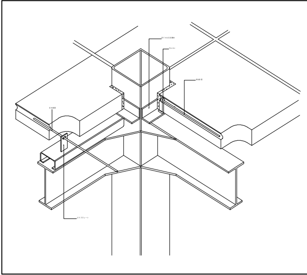
ヤネ1カP-8
