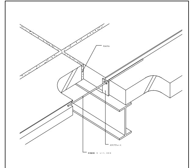
ヤネ1カP-1
