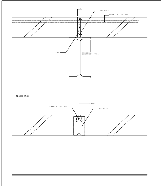
ヤネ1カ-4
