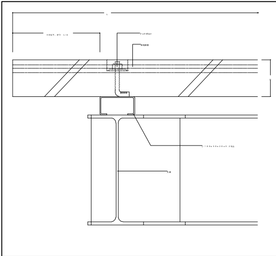
ヤネ1カ-10
