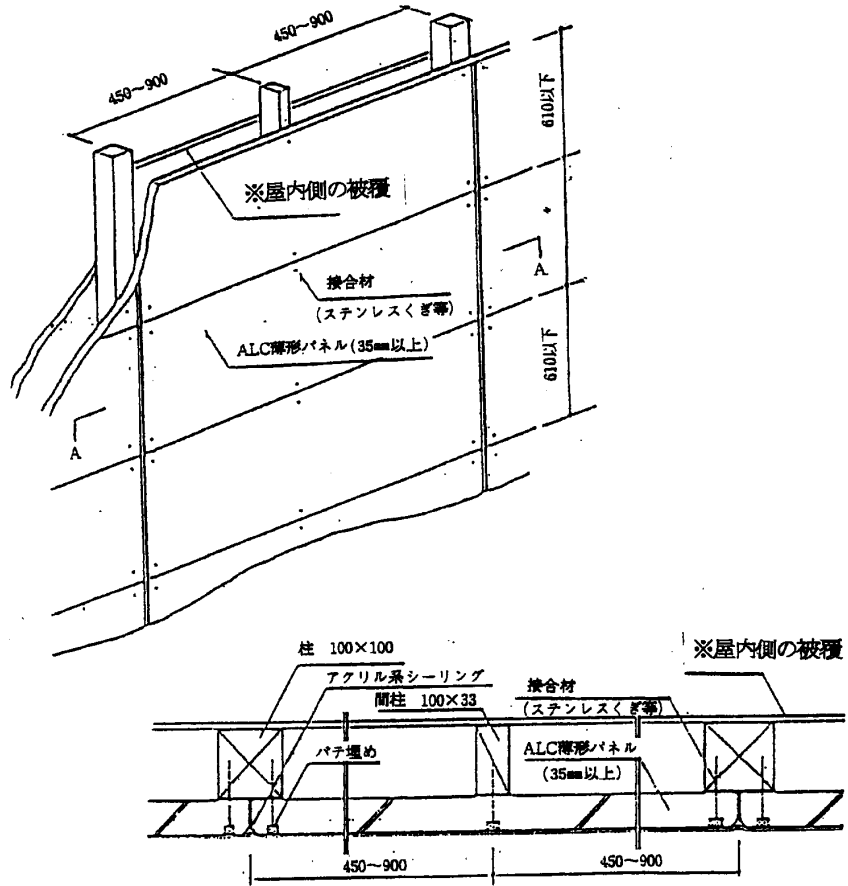
A-A 断面図
